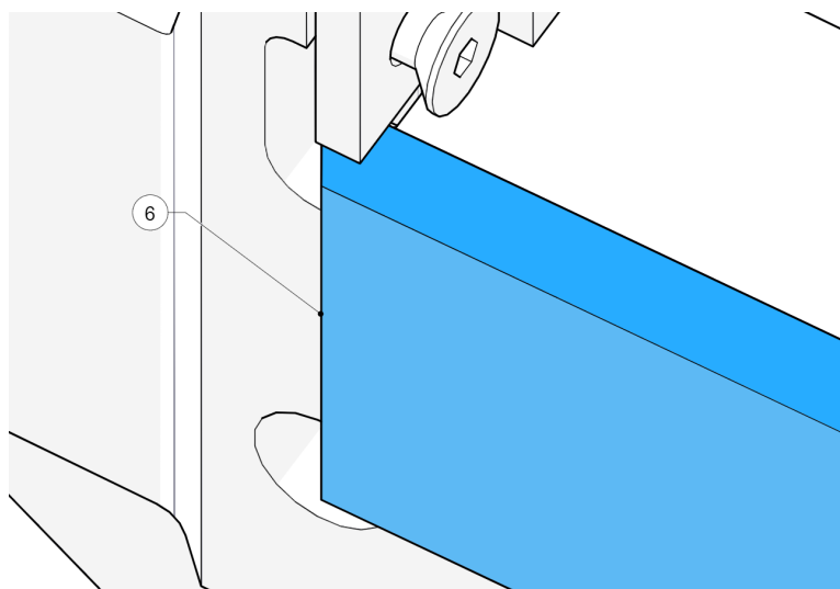
Figure 63 - Enclume dans le siège vertical
