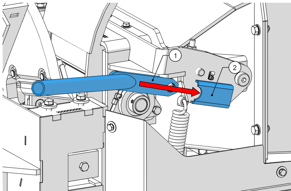
Figure 42 - Tension du ressort du rouleau d'alimentation
