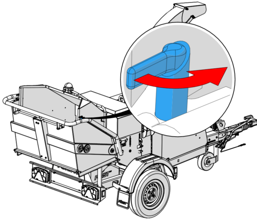
Figure 30 - Loquet de verrouillage du plateau de trémie
