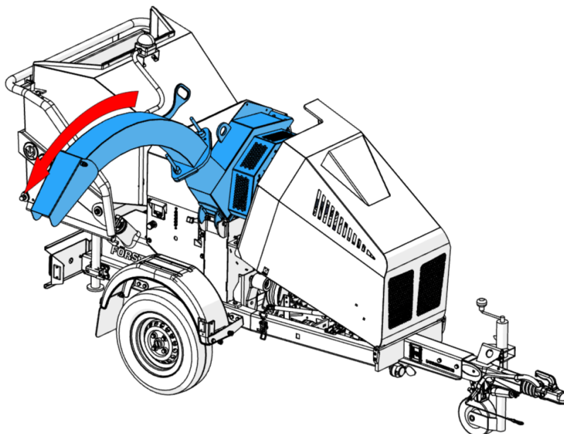
Figure 47 - Ouvrez le couvercle de la chambre de broyage
