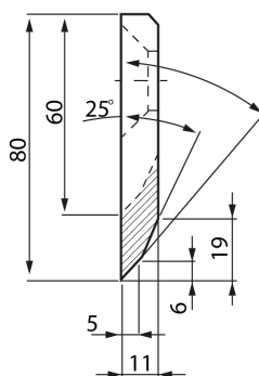
Figure 56 - Limite d'usure d'affûtage de la lame : 80 mm à 60 mm
