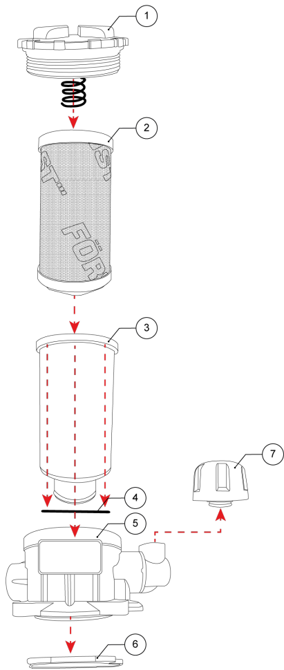
Figure 67 - Filtre à huile hydraulique
