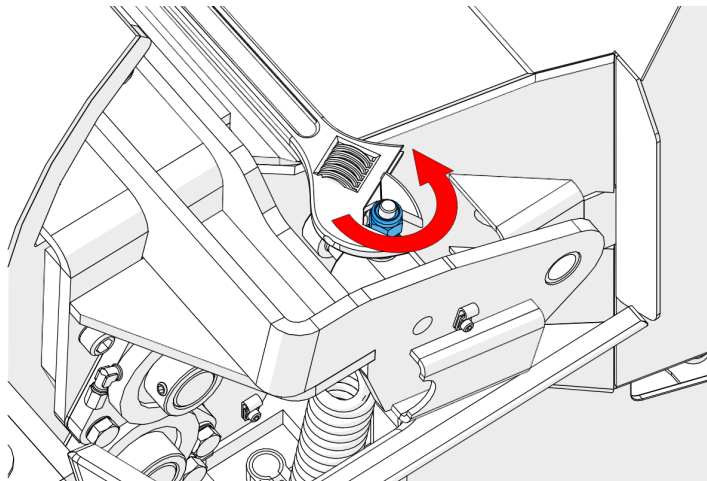
Figure 41 - Ressort cintre écrou
