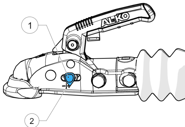
Figure 23 - Témoin d'usure de l'attelage de remorque
