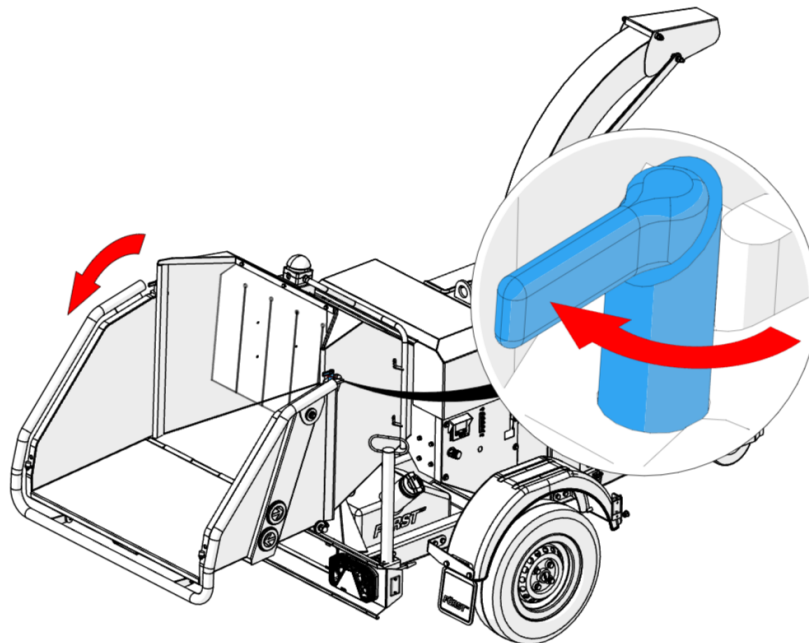
Figure 31 - Plateau de trémie verrouillé en position basse
