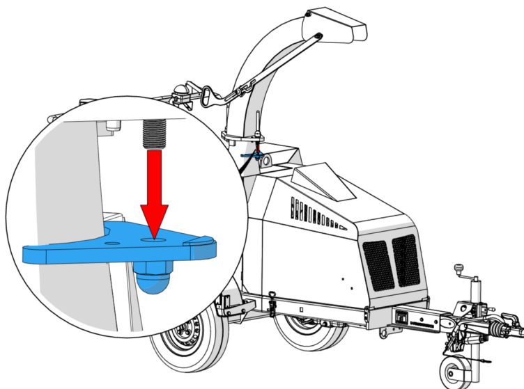
Figure 27 - Retirer le collier et l'écrou
