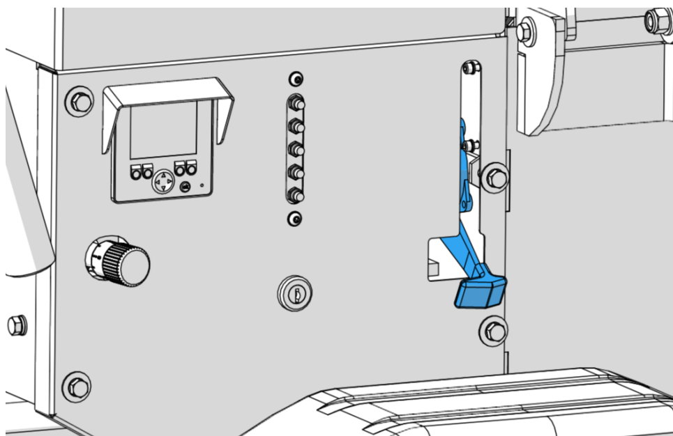
Figure 34 - Position maximale de l'accélérateur
