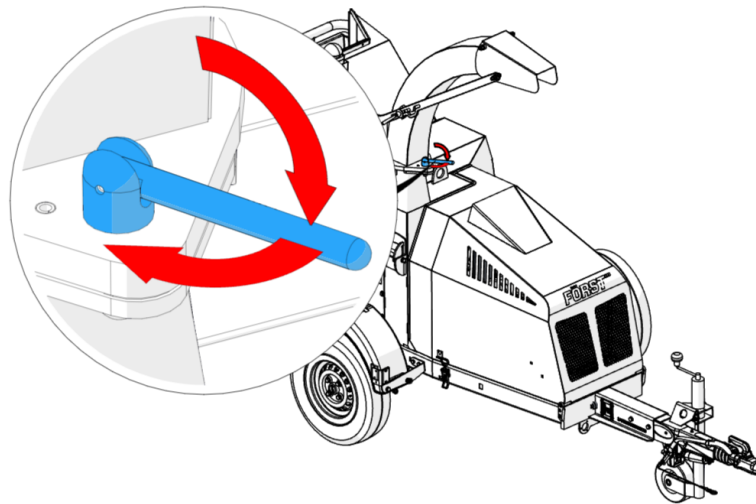
Figure 26 - Rotation de la goulotte
