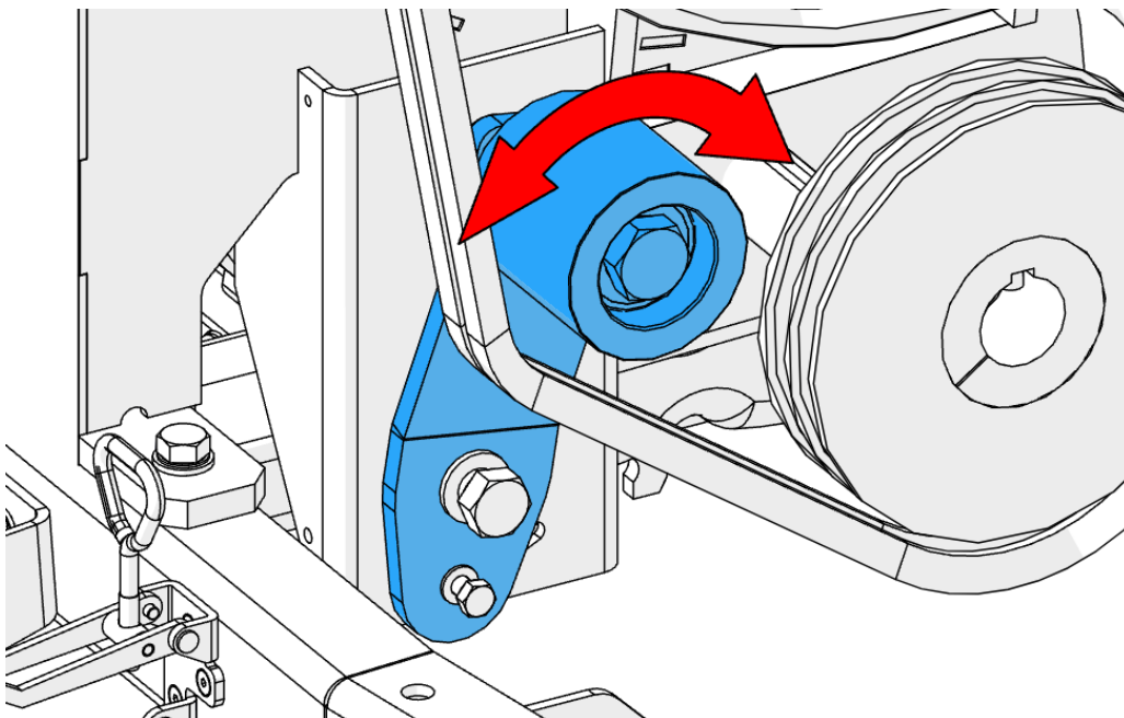
Figure 66 - Tendeur de courroie trapézoïdale
